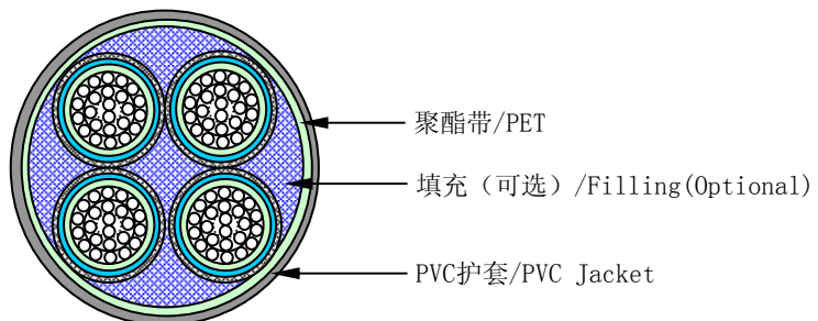
图二：程控交换机用局用电缆（ADSL电缆）结构图
