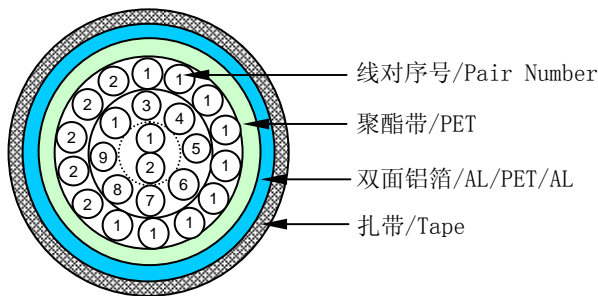
图一：24对单位缆结构图
